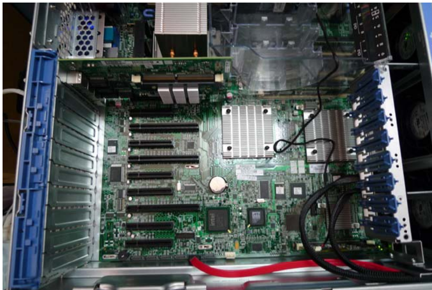
圖 167. 伺服器內部主機板
